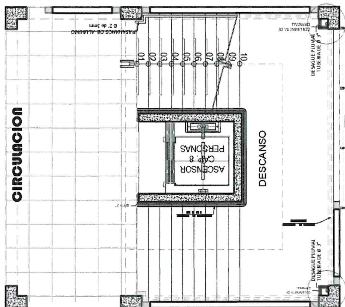
PRIMERA PLANTA - MODULO 03
