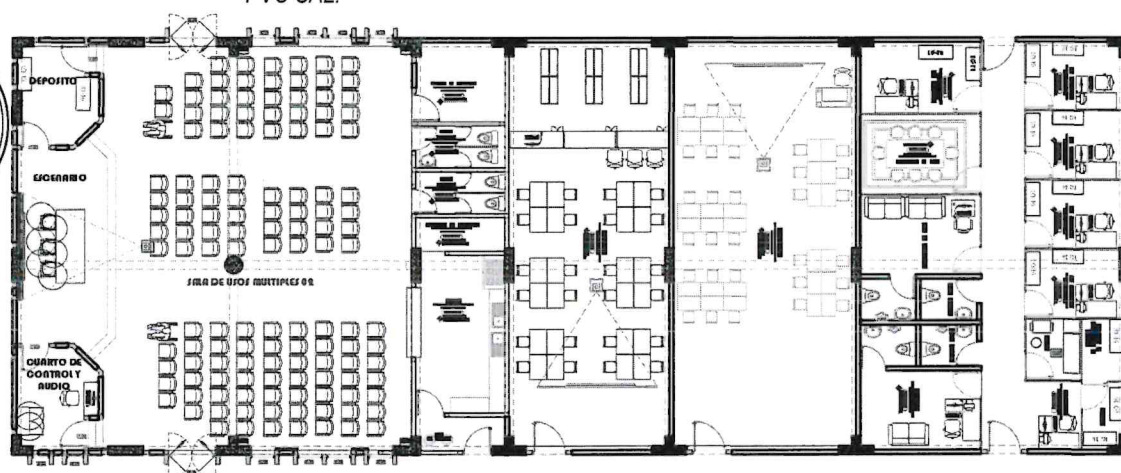
PRIMERA PLANTA - MODULO 03 Escala 1:75
