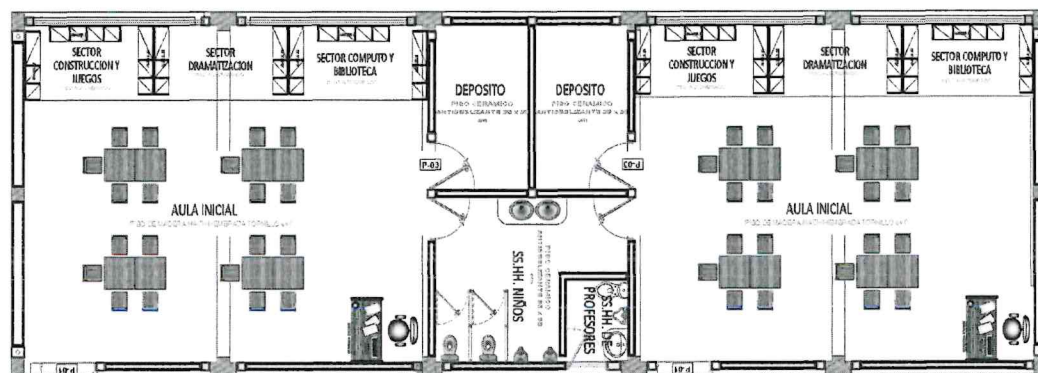
PRIMERA PLANTA - MODULO 08 E.E. 1279
