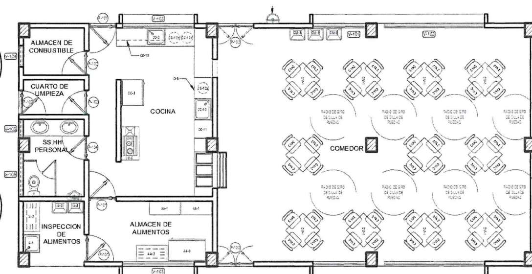
PRIMERA PLANTA - MODULO 09 25.04.79
